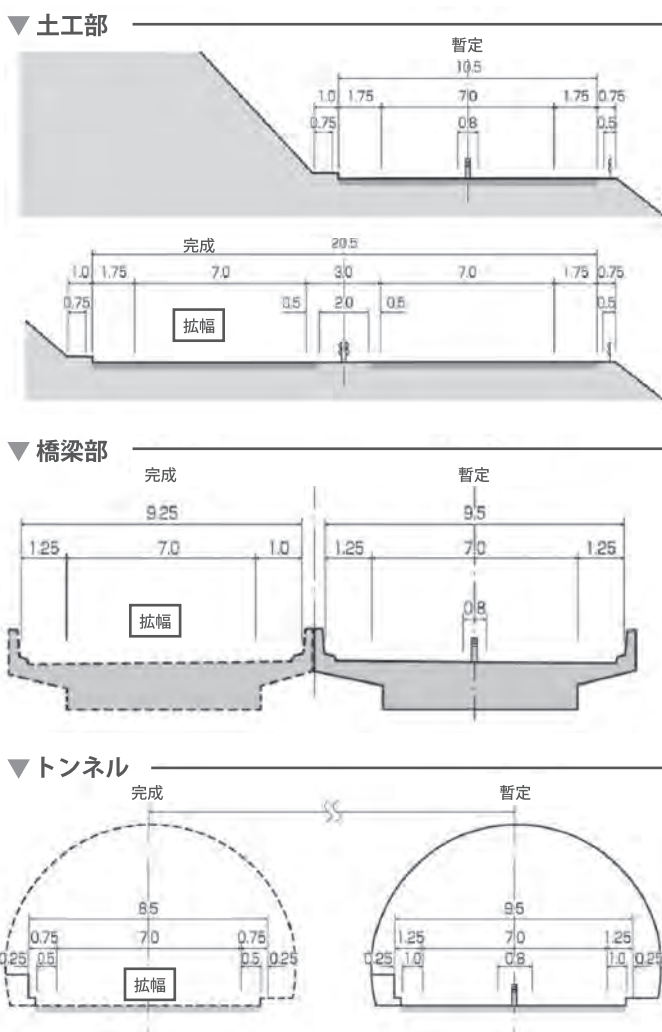
【標準断面図】
